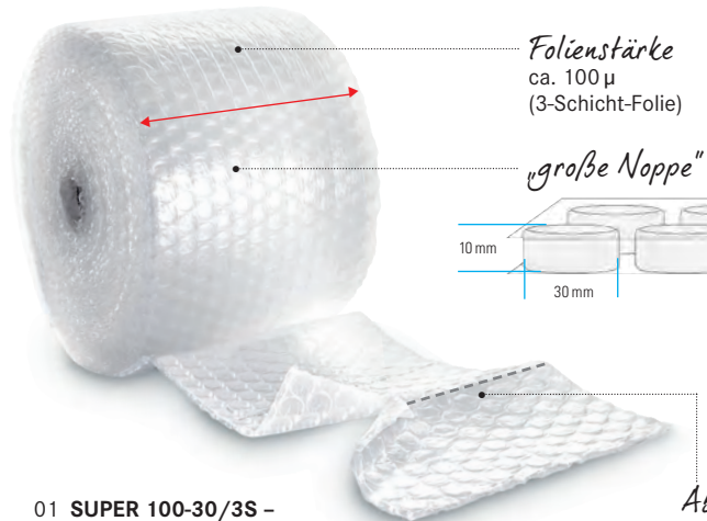
01 SUPER 100-30/3S – abrisssperforiert „Luftpolsterfill“
