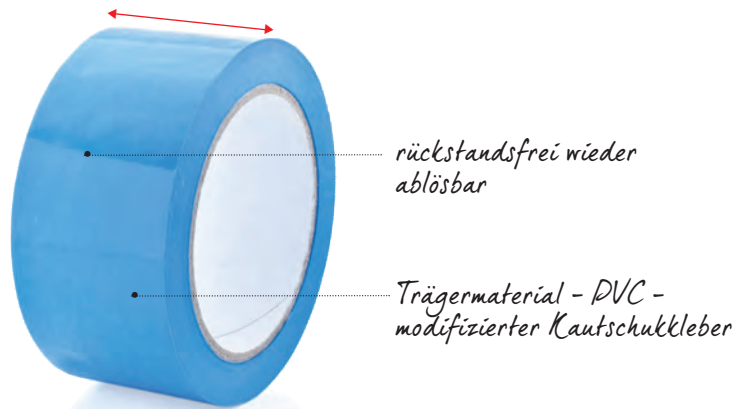
01 Spezial-Klebeband QR (quick release)
