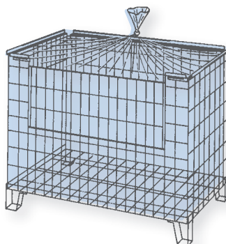
04 Kompletthaube (als Einstellhaube, am Beispiel Euro-Gitterbox)
