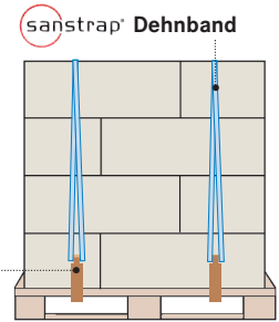
Vertikale Palettensicherung in Verbindung mit sanstrap® Dehnbändern
